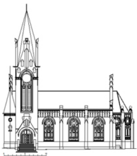
Рис.1. Церковь Св. Павла. Арх. Г.Р. Юнгхендель. Владивосток. 1908: а – чертеж автора; б – почтовая открытка [5]
