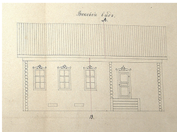
Рис. 6.1. Главный фасад дома В.С. Кузнецова
