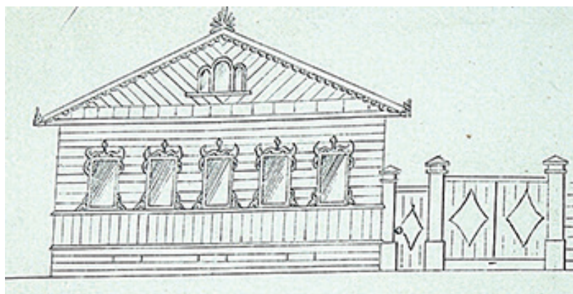
Рис. 8.2. Фасад дома по линии АВ 9
