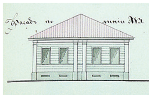
Рис. 5.3. Фасад дома по линии АВ 6
