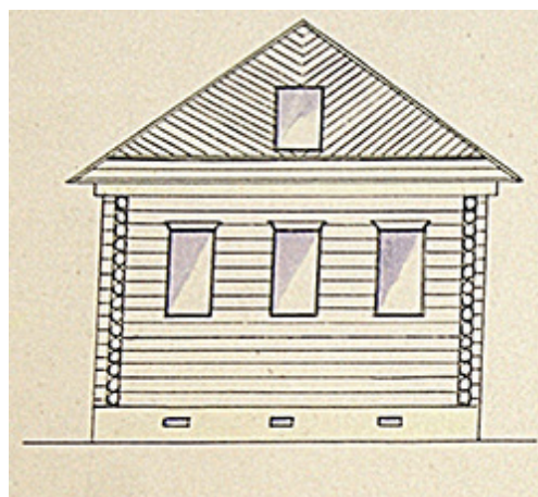
Рис. 4.3. Фасад дома по линии АВ 5
