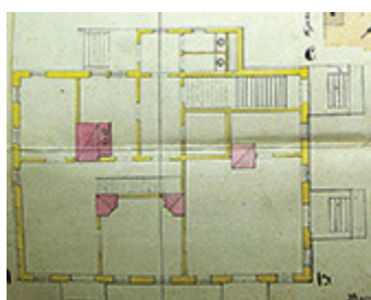
Рис. 14.2. План 1-го этажа дома А.И. Чуриловой 15
