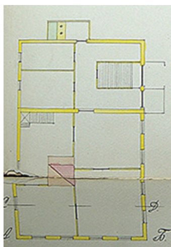
Рис. 12.2. План дома Ф.Я. Разанова 13
